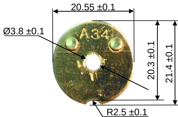
REF.23 - P. N° 14-A34 THROTTLE SHUTTER PAPILLON CARBURATEUR
