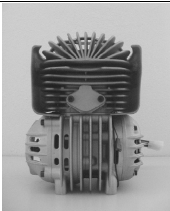
BILDE AV MOTOR (FORFRA)
