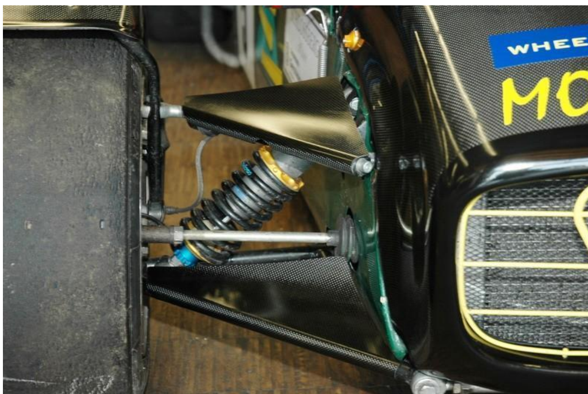
Figur 2 viser bærebri «vinger» for biler med klassisk karosseri iht pkt.12 i Teknisk reglement for Seven Racing.
