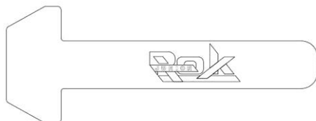
DIMA CONTROLLO COLLETTORE MANIFOLD CONTROL TEMPLATE
